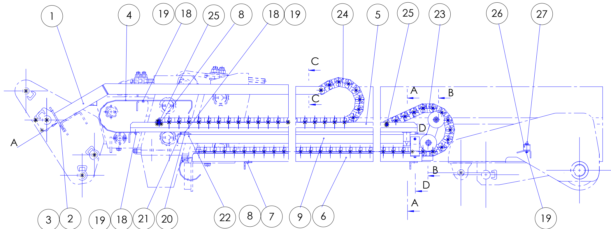
LEIKK B--B
