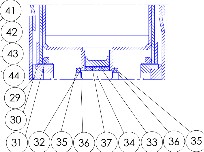
LEIKKAUS A----A
